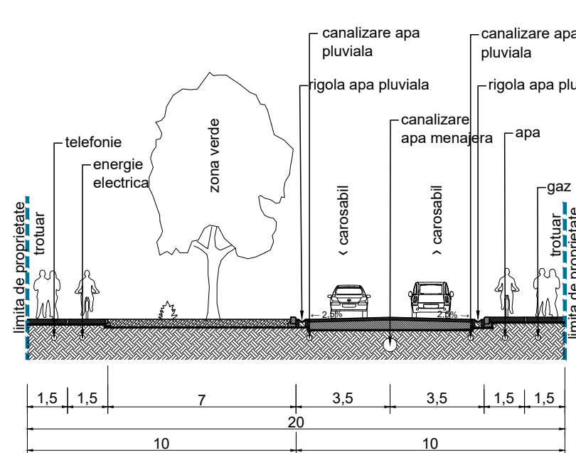
Profil transversal 3-3
