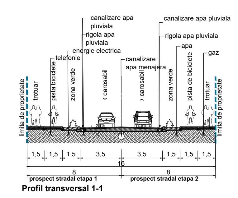
Profil transversal 1-
