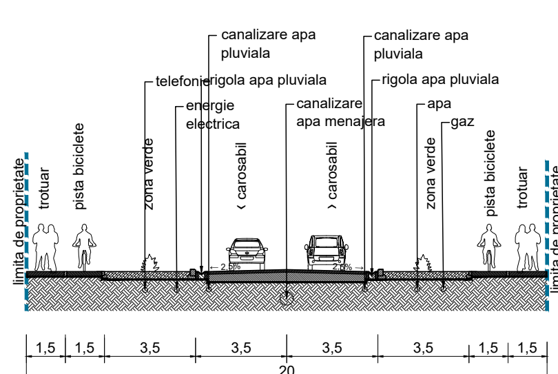
Profil transversal 2-2
